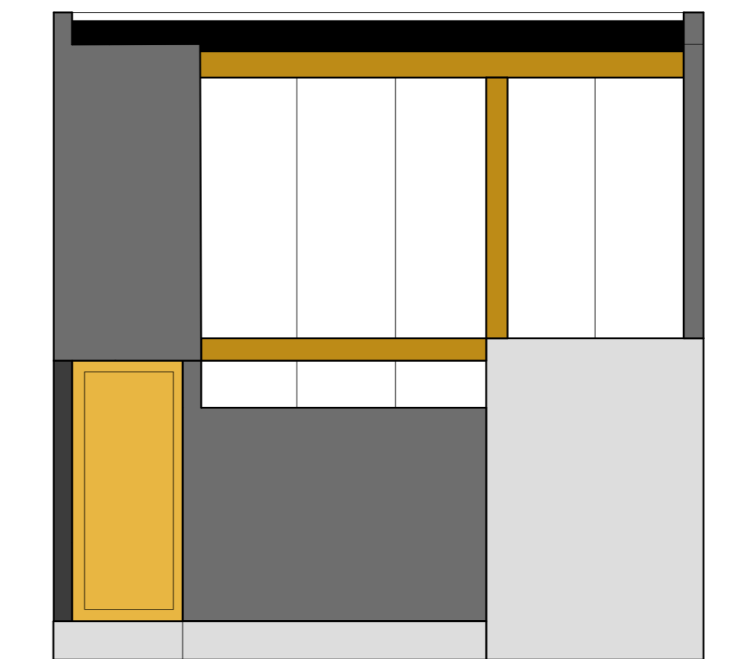
FACHADA ESCALA 1:50
